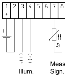
Type -Px, -PTx (2-wire)
