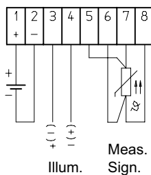
Type -PxL4, -PTxL4 (4-wire)
