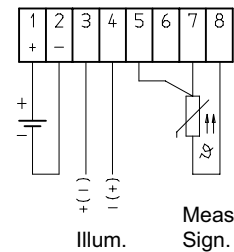
Type PxL3, Type PTxL3 (3-wire)
